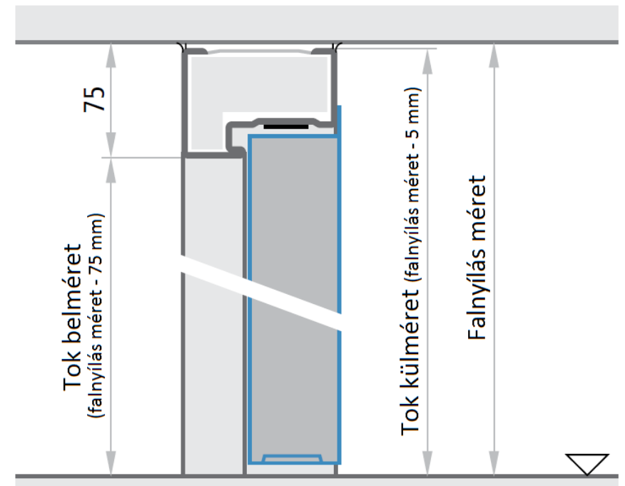
Függőleges metszet
