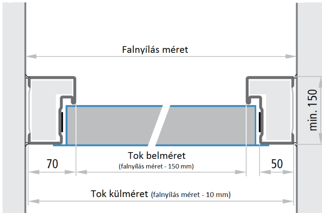
Vízszintes metszet
